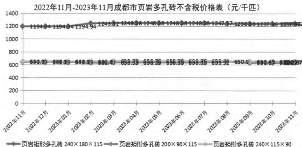
2022 年 11 月 -2023 年 11 月成都市豆石不含税价格表 (元 / m 3 )
