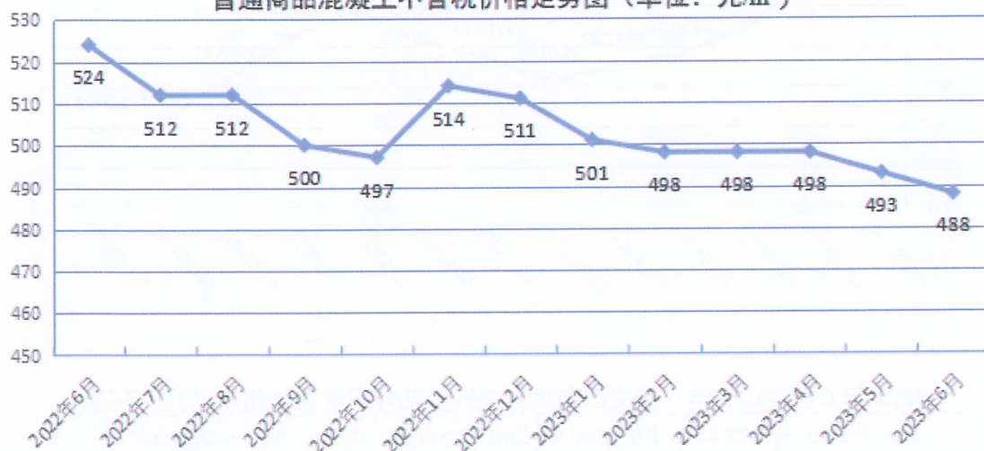
2022年6月-2023年6月成都市商品混凝土C30含三环里以内工地运输费 普通商品混凝土不含税价格走势(单位:元/m³)
