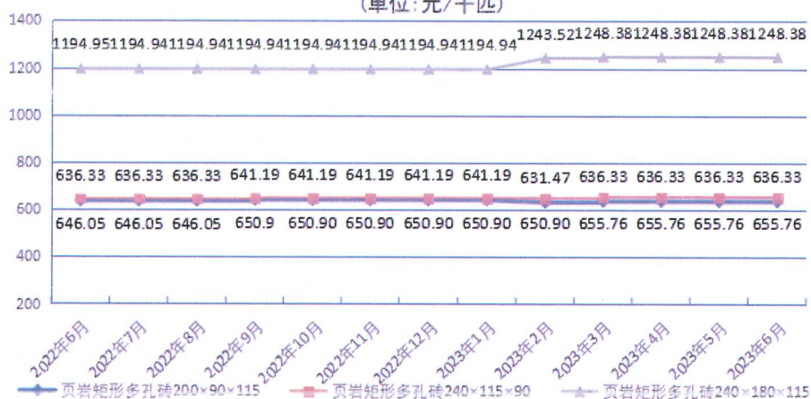
2022年6月-2023年6月成都市页岩矩形多孔砖不含税价格走势 (单位:元/千匹)
