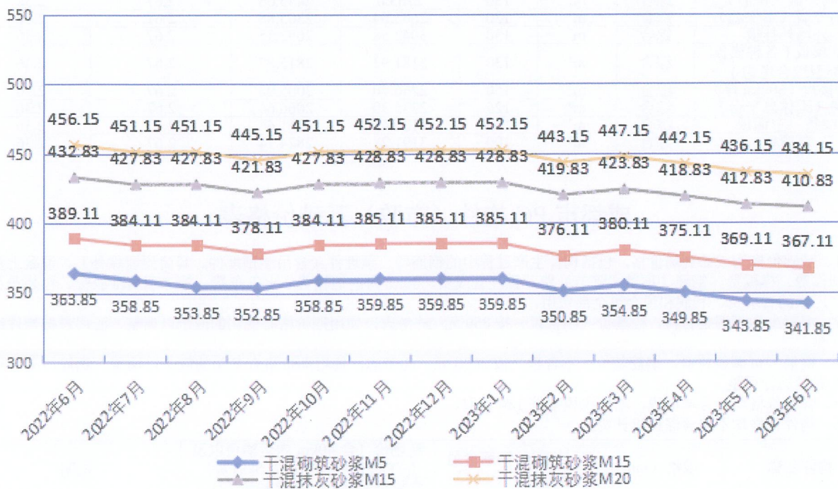
2021年6月-2023年6月成都市砂浆不含税价格走势图(单位:元/m 3 )
