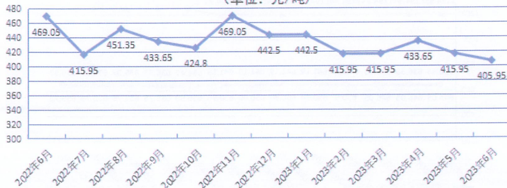
2022年6月-2023年6月成都市水泥PO42.5R不含税价格走势 (单位:元/吨)
