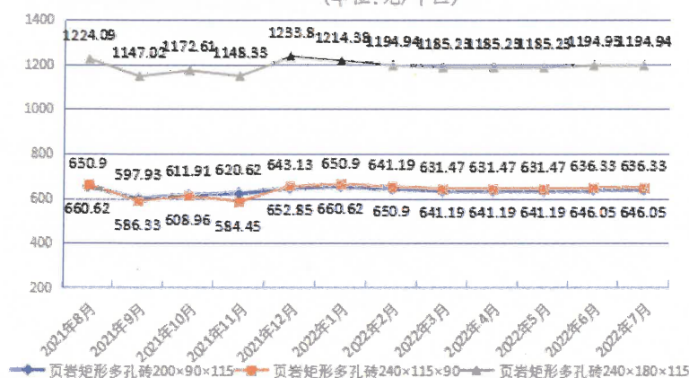
2021年8月-2022年8月成都市页岩矩形多孔砖不含税价格走势 (单位:元/千匹)
